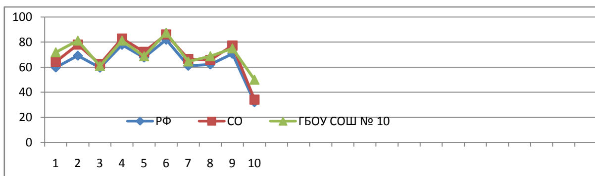
Выполнение заданий ВПР по обществознанию в 8 классе
