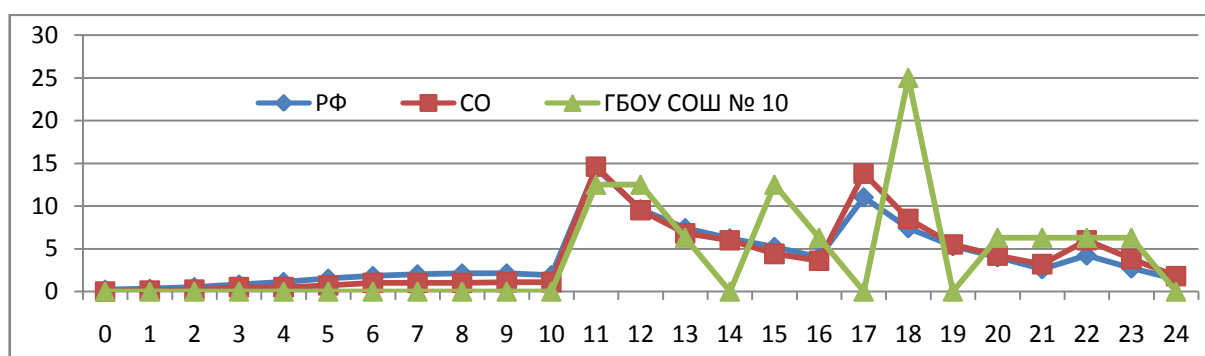
Распределение участников ВПР по обществознанию 8 классов по сумме полученных первичных баллов
