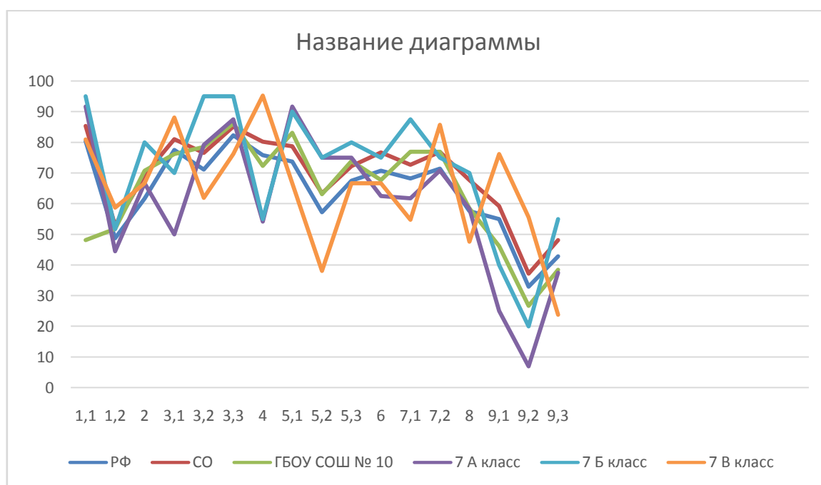
Выполнение заданий ВПР по обществознанию в 7-х классах
